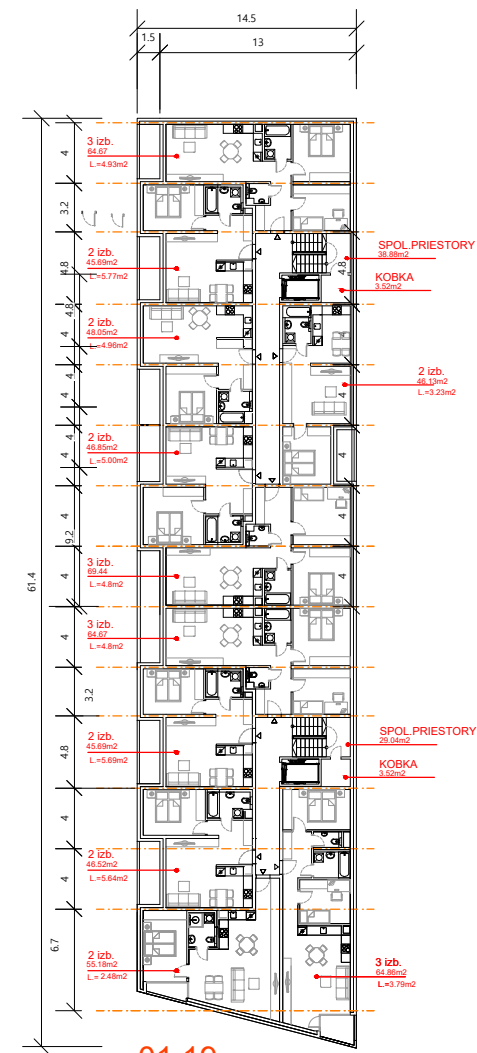
01.19 TYP B 2-5. NP
