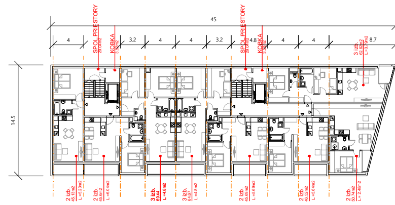
01.19 TYP A 2-5. NP
