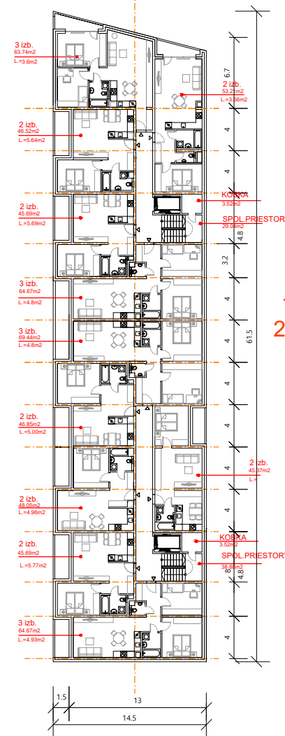
01.19 TYP C 2-5. NP
