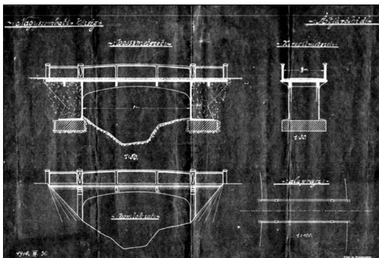
Projekt prechodného mostu v Trnave – rez priečný, pozdĺžny, pohľad pôdorys 30. 7. 1916 – Pittel és Brausewetter 39x 56,5 (Štátny okresný archív v Trnave)
