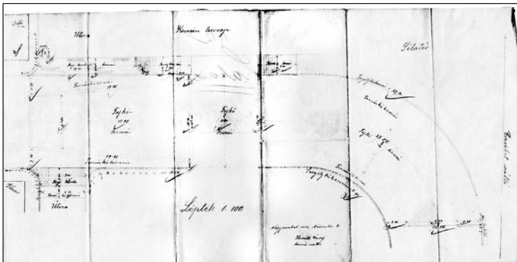
Plán dláždenia (úsek čiastkový) poloha na Ulici A. Žarnova – pri dnešnom Okresnom dome, pôdorys m 1: 100, Trnava, 9. 11. 1912 Horváth József, 34 x 66, orientačné body – Promenáda setatér, Glaser, Braun (Štátny okresný archív v Trnave).
