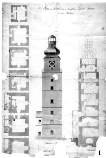
Nákres mestskej veže z pohľadu od Štefánikovej ulice, 1864.
