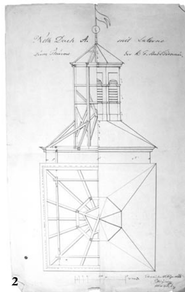
2 – 7 Rozličné nákresy a návrhy strechy mestskej veže z rokov 1864 – 1875.
