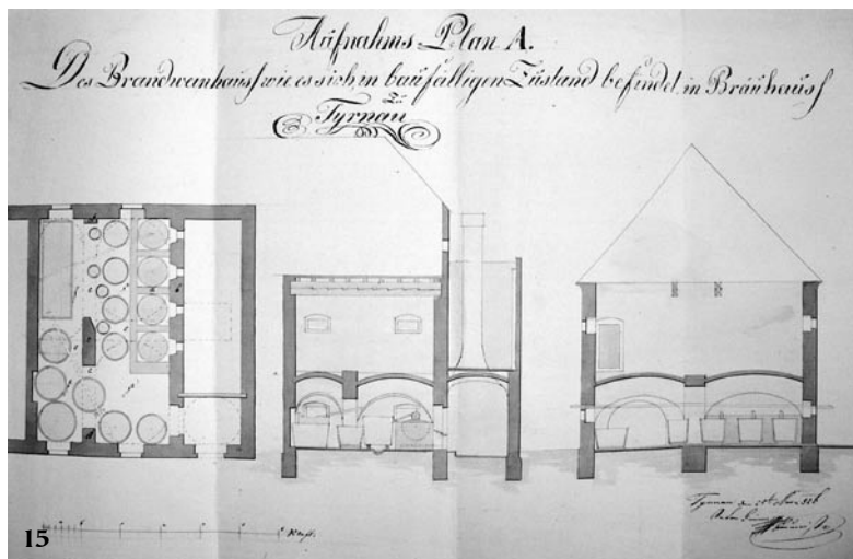
Plán schátranej pálenice v budove pivovaru.
