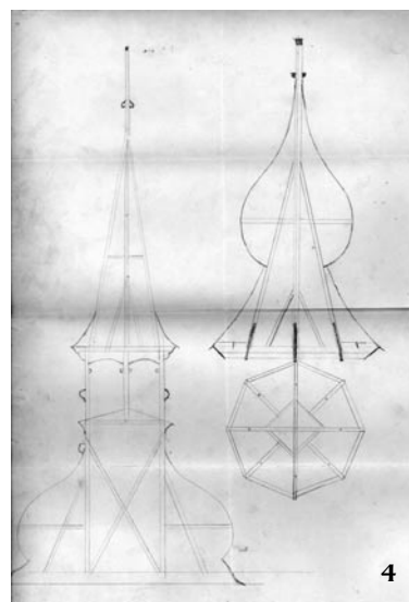
2 – 7 Rozličné nákresy a návrhy strechy mestskej veže z rokov 1864 – 1875.
