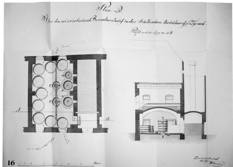
Plány prestavby pivovarskej pálenice.
