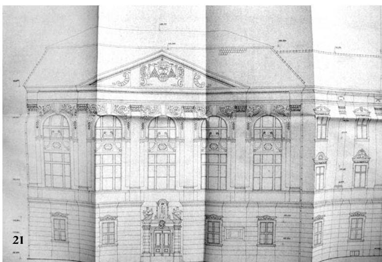
Zameranie fasády kasární kpt. Jána Nálepku, sála Marianum.
