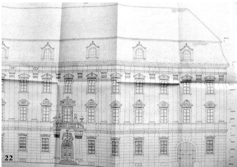
Zameranie fasády kasární kpt. Jána Nálepku, Šľachtický konvikt.
