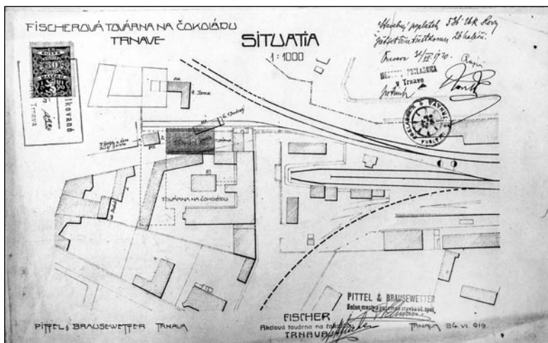
Výkres situácie z roku 1919 k výstavbe skladu. Vidno na nej postupne zanikajúcu Mesačnú ulicu (zdroj: ŠOKA - MÚ Trnava - technické oddelenie - fascichel Figaro)
