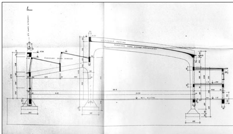
Rez novou zlievarňou (zdroj: Štátny archív v Trnave, ONV Trnava I – administratíva, kr. 204, inv. č 27 499, – Plány prístavby zlievarne firmy Kovosmalt, n. p. Trnava, 1948)
