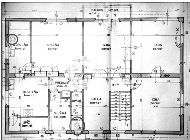
Vila Dušana Jurkoviča – projekt z roku 1938, Štátny archív v Trnave, I/2 Okresný úrad Trnava, Administratívne spisy; šk. 374, inv. č. 8 266/41
