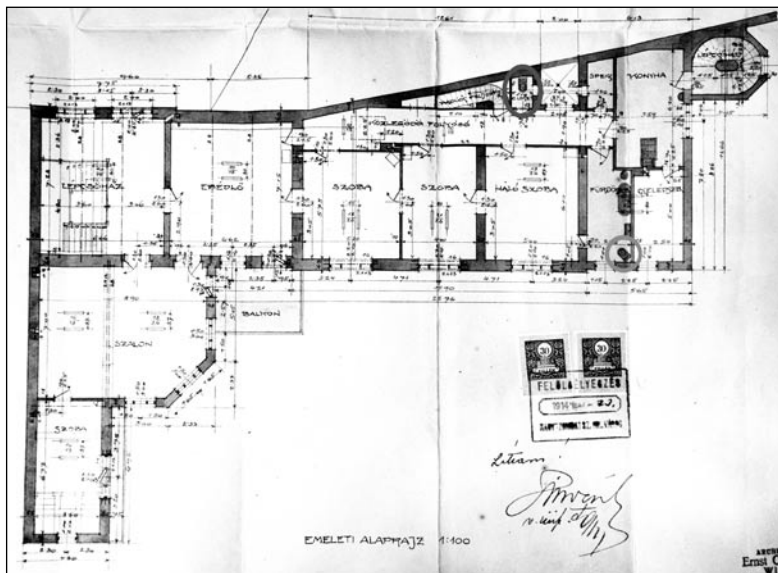
Koppelova vila – projekt prestavby z roku 1913, Štátny archív v Trnave, II/19 Magistrát mesta Trnava Technický odbor; šk. 4, inv. č. III/54
