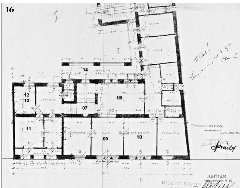
Plán riaditeľského bytu z roku 1920 pred stavbou bytového domu na Emmerovej 11 (dnes A. Žarnova 51), zdroj: Štátny archív v Trnave
