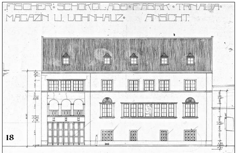
Návrh priečelia trojpodlažného bytového domu a obchodu s výrobkami továrne Fischer, ktorý mal byť na prízemí a vo dvorovej časti, 1920, zdroj: Štátny archív v Trnave
